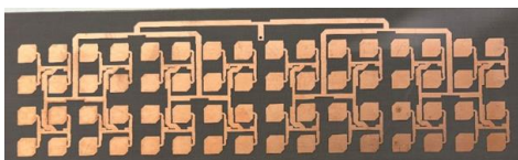
図1 試作したパッチアレーアンテナ基板
