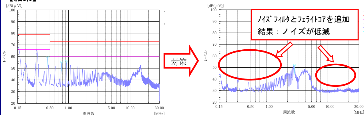
図 1 実際の機器のノイズ対策（左図：対策前 右図：対策後）
