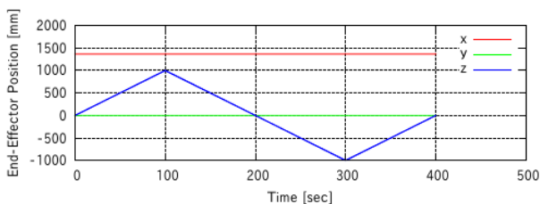
図 8 手先位置の目標値(縦方向動作)
