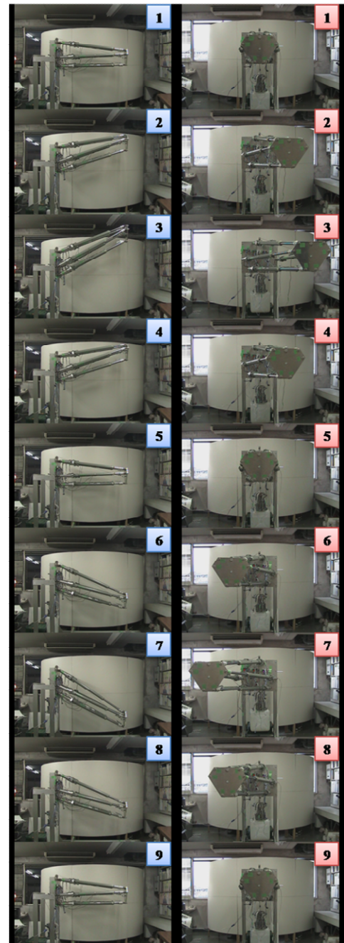
図 7 マニピュレータ動作の様子 (左:縦方向動作, 右:横方向動作)
