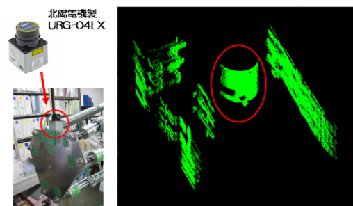
図 16 (左) 測域センサ, (右) 形状計測結果
