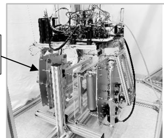
開発中のドローン吊り下げ補修ロボット
