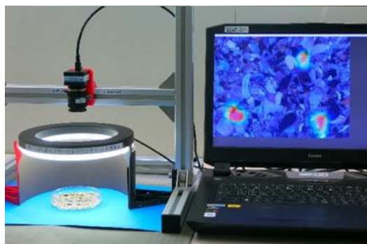
ハマグリの稚貝検出装置
